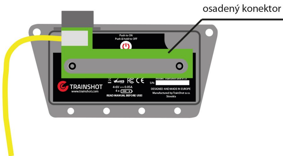
Zadná strana osadeného konektora
